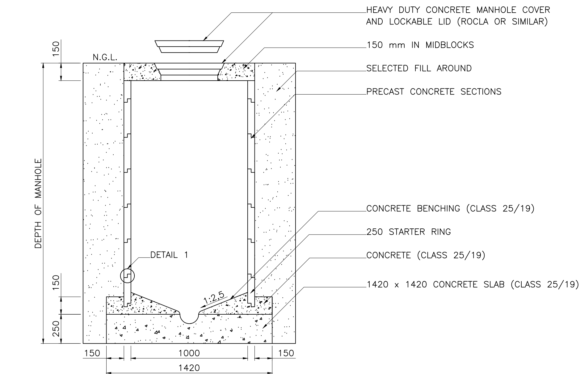
SECTION A-A
